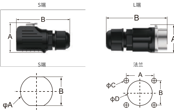
尺寸图 Dimension drawing
