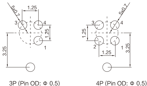
M5母头, PCB型, 前锁, 屏蔽
