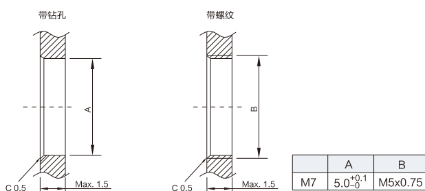
M5母头, 面板式, 焊接型, 后锁连接器
