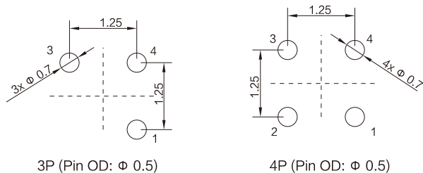
M5母头, PCB型, 前锁
