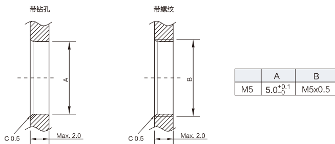
M5公头连接器
